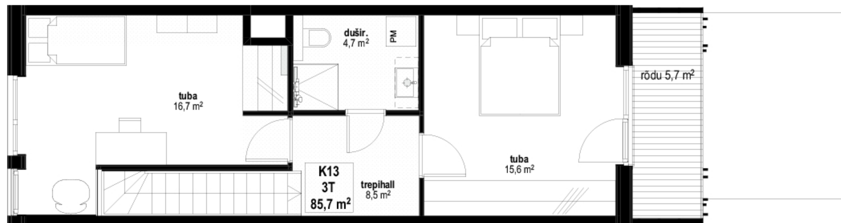
3. korrus
